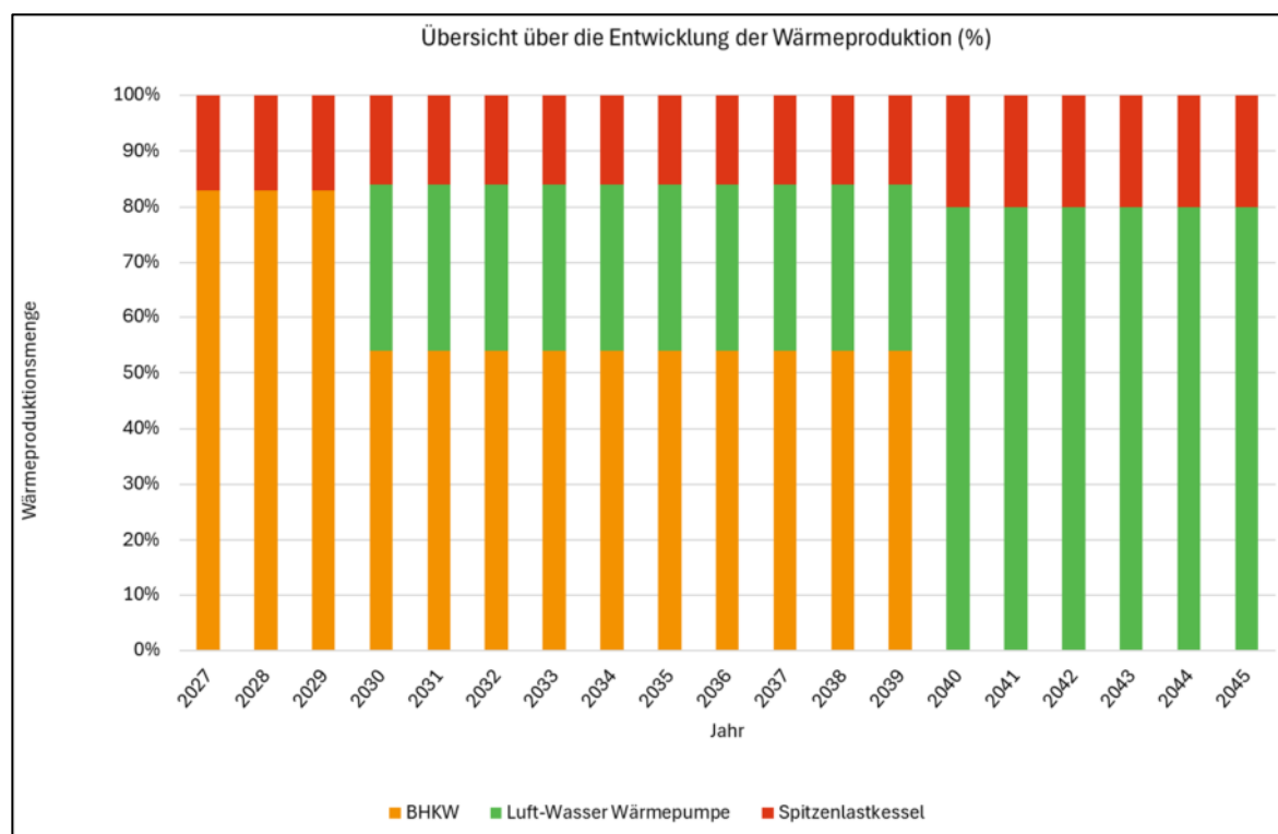
Abbildung 18: Verteilung der Wärmeproduktion auf die Wärmeerzeuger
