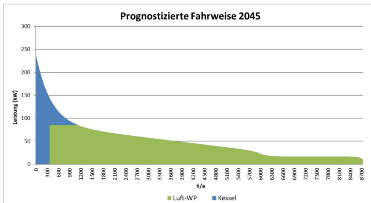
Abbildung 21: Jahresdauerlinie nach Maßnahmenpaket 3
