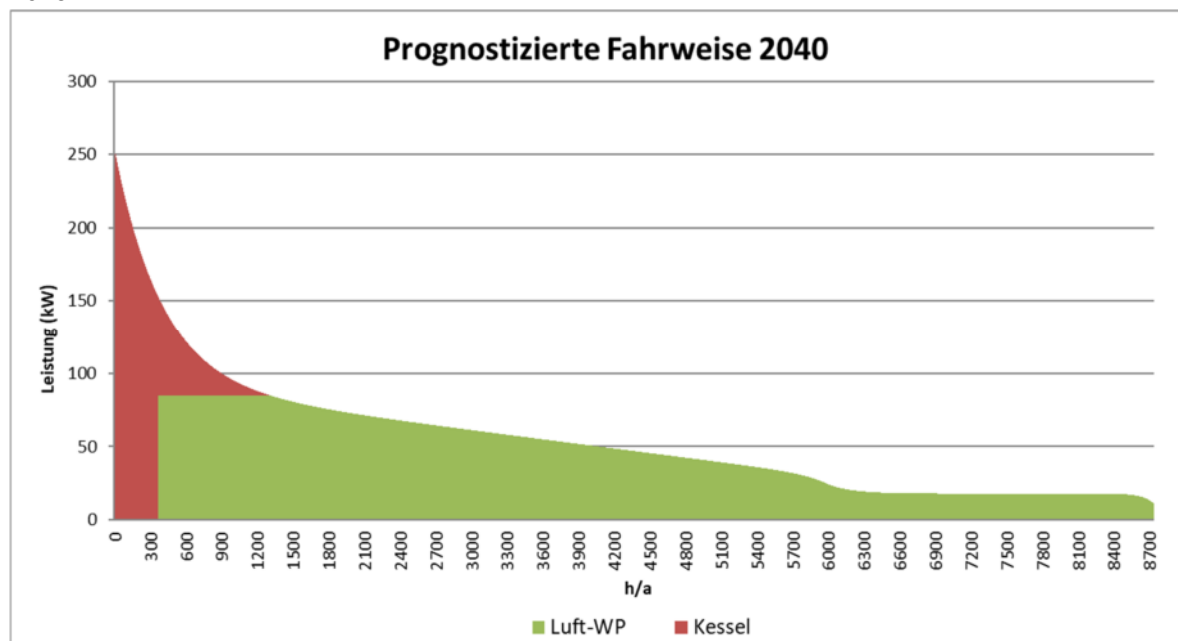
Abbildung 20: Jahresdauerlinie während Maßnahmenpaket 2
