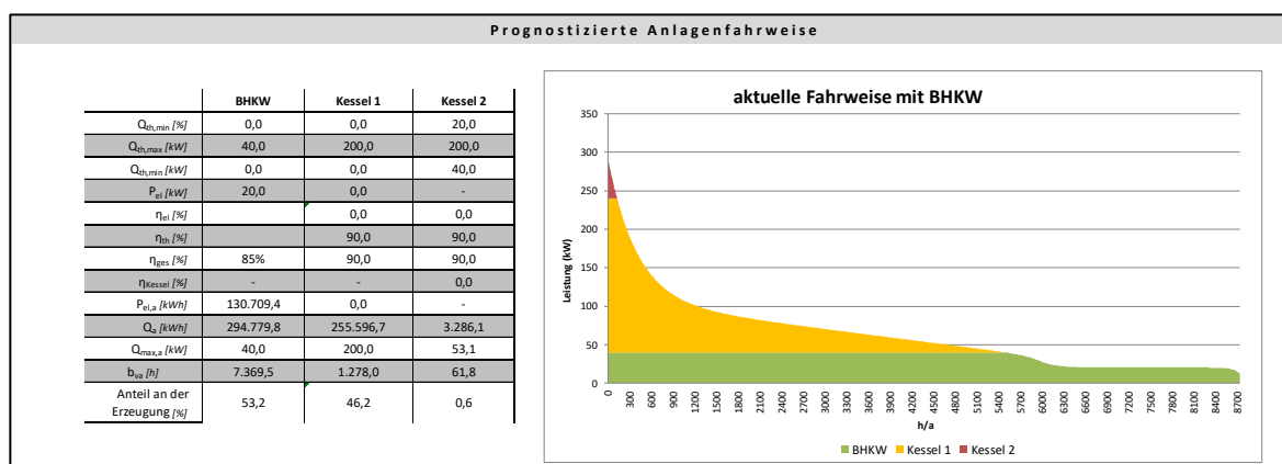
Abbildung 7: Anlagenfahrweise im IST-Zustand
