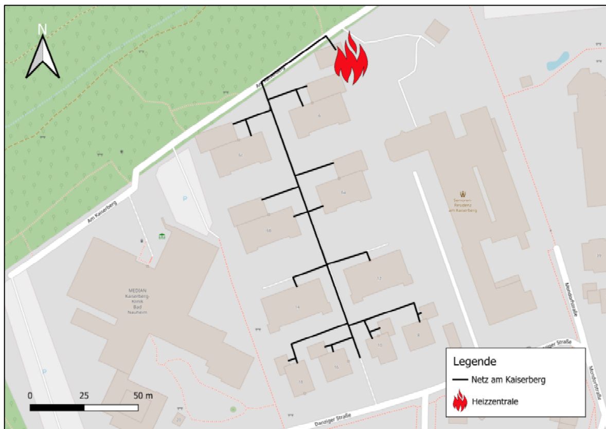
Abbildung 6: Darstellung Heizzentrale
