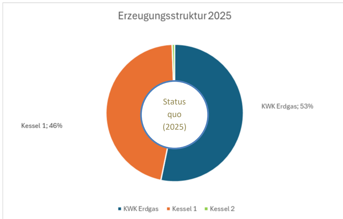
Abbildung 8: Erzeugerstruktur im IST-Zustand
