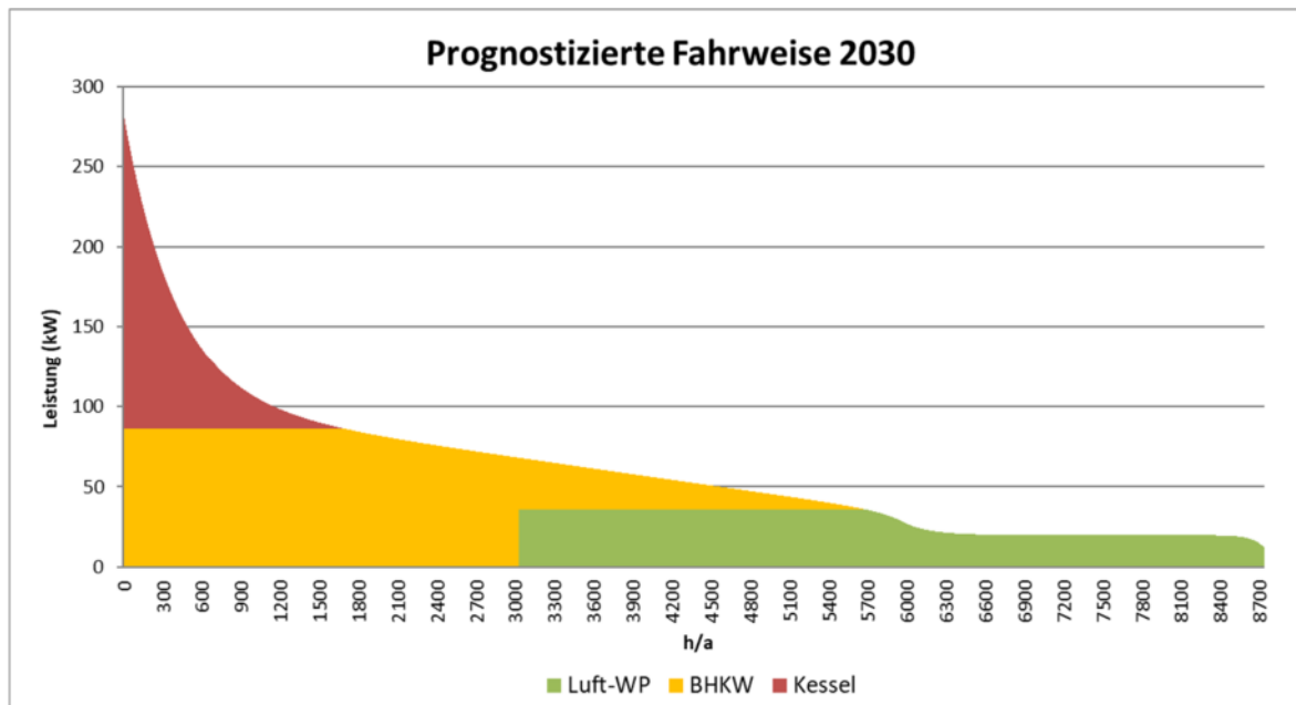
Abbildung 19: Prognostizierte Fahrweise 2030
