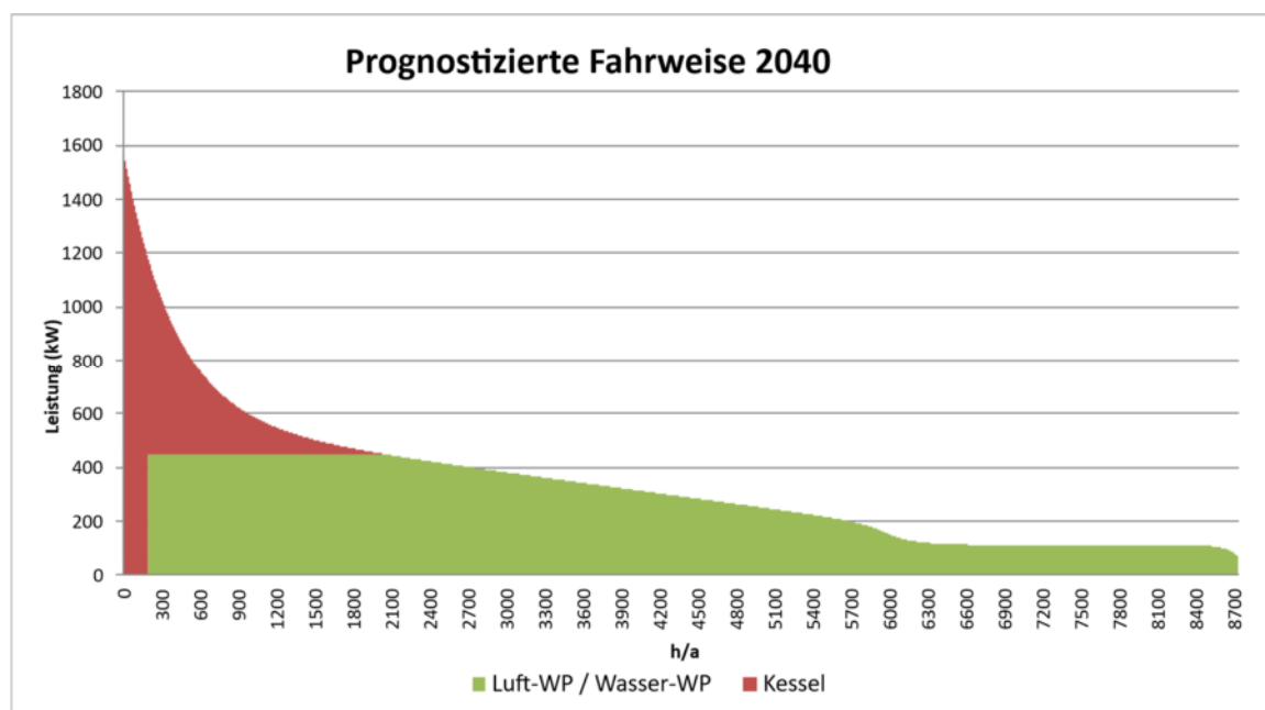
Abbildung 21: Jahresdauerlinie während Maßnahmenpaket 2
