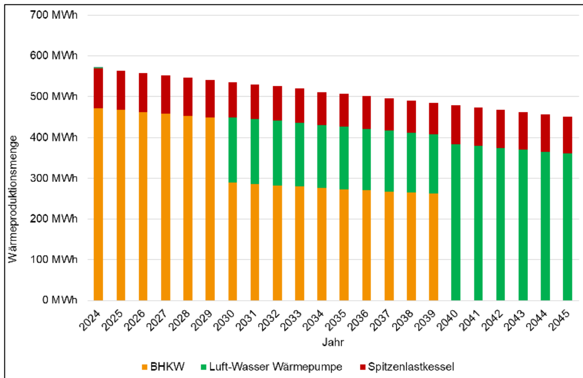
Abbildung 17: Wärmeproduktionsmengen im Zeitverlauf
